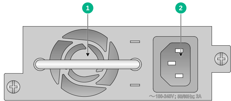
图A-7 交流电源模块外观
