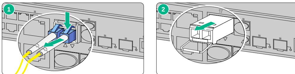
图4-4 拆卸光接口模块示意图
