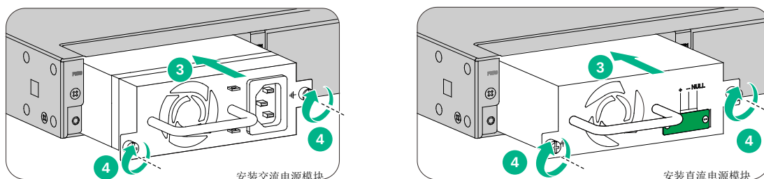
图2-11 安装电源模块
