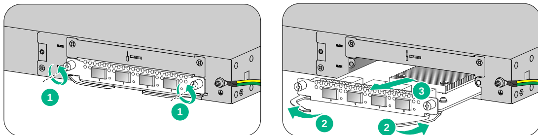
图4-2 拆卸接口模块
