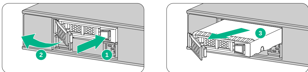
图2-15 拆卸硬盘
