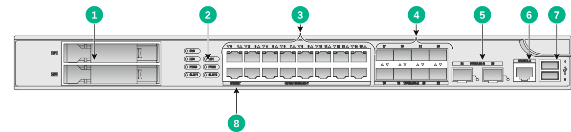
图A-3 设备前视图
