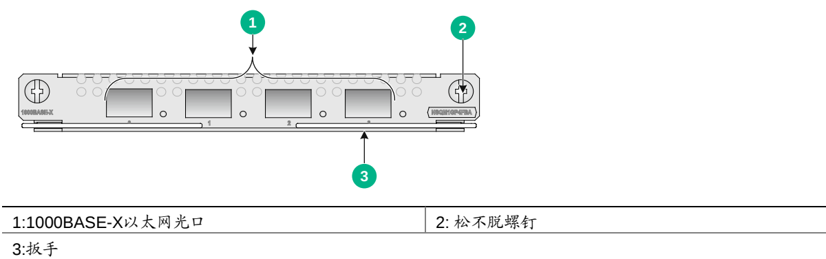
图A-6 NSQM1GP4FBA 接口模块正视图
