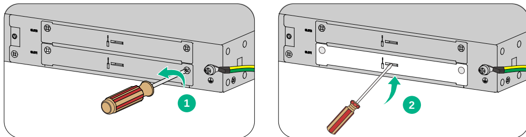
图2-12 拆卸假面板
