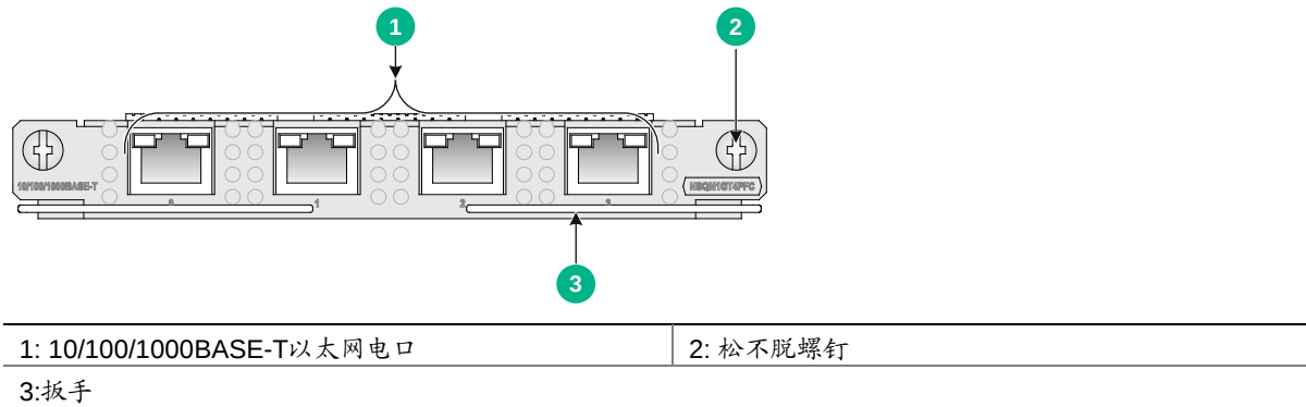
图A-5 NSQM1GT4PFC 接口模块正视图
