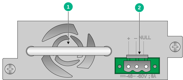
图A-8 直流电源模块外观
